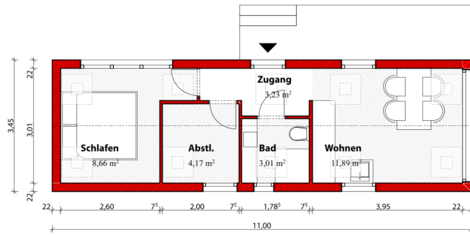
Grundriss
