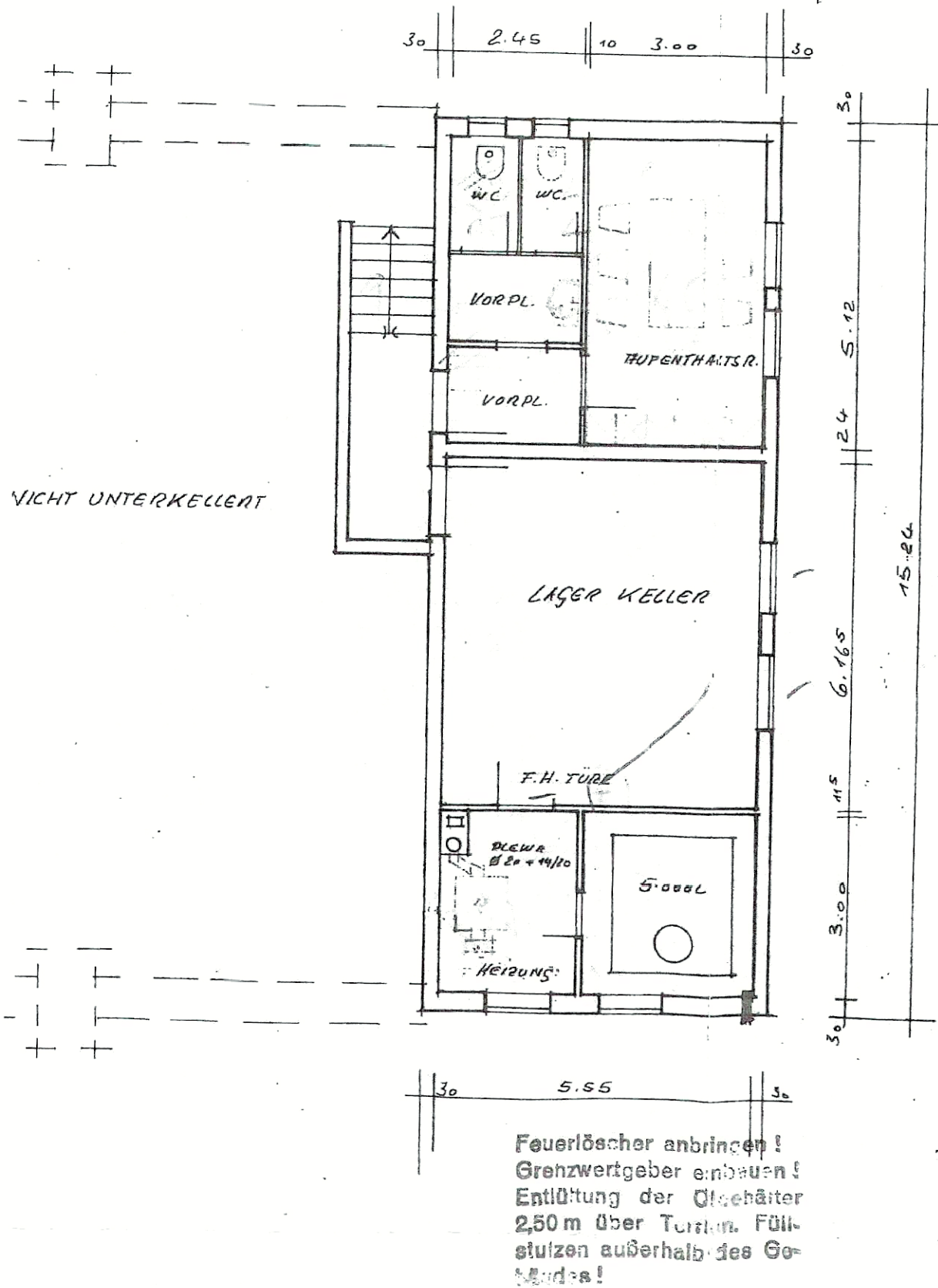
Untergeschoss Bestand
