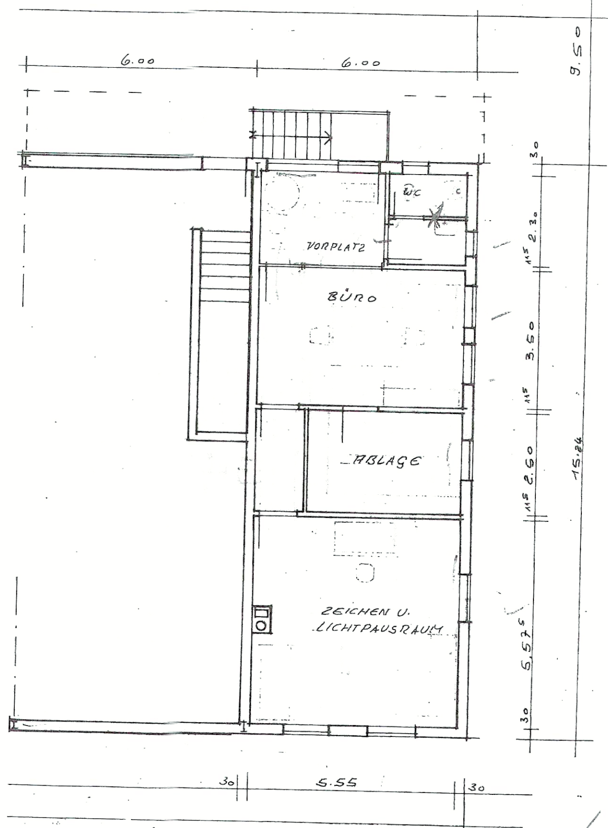
Erdgeschoss Bestand
