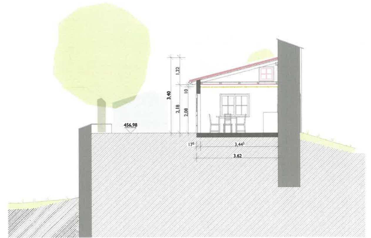
S3 quer 1:100
