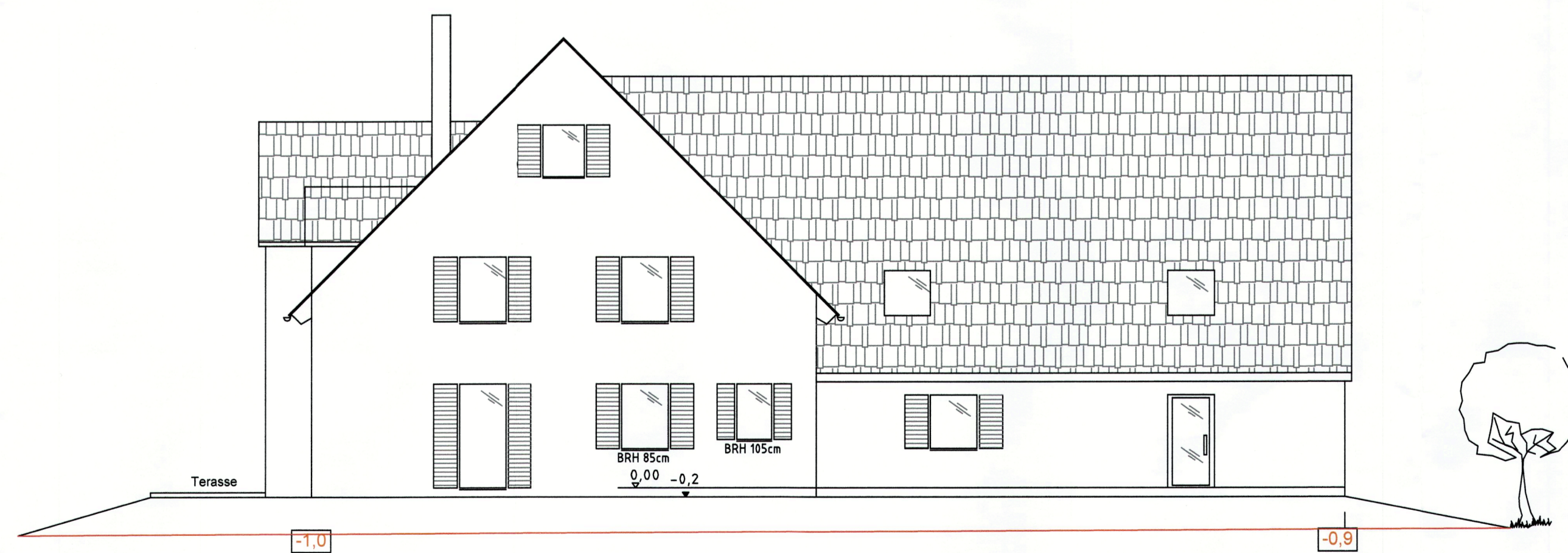
SÜDANSICHT
